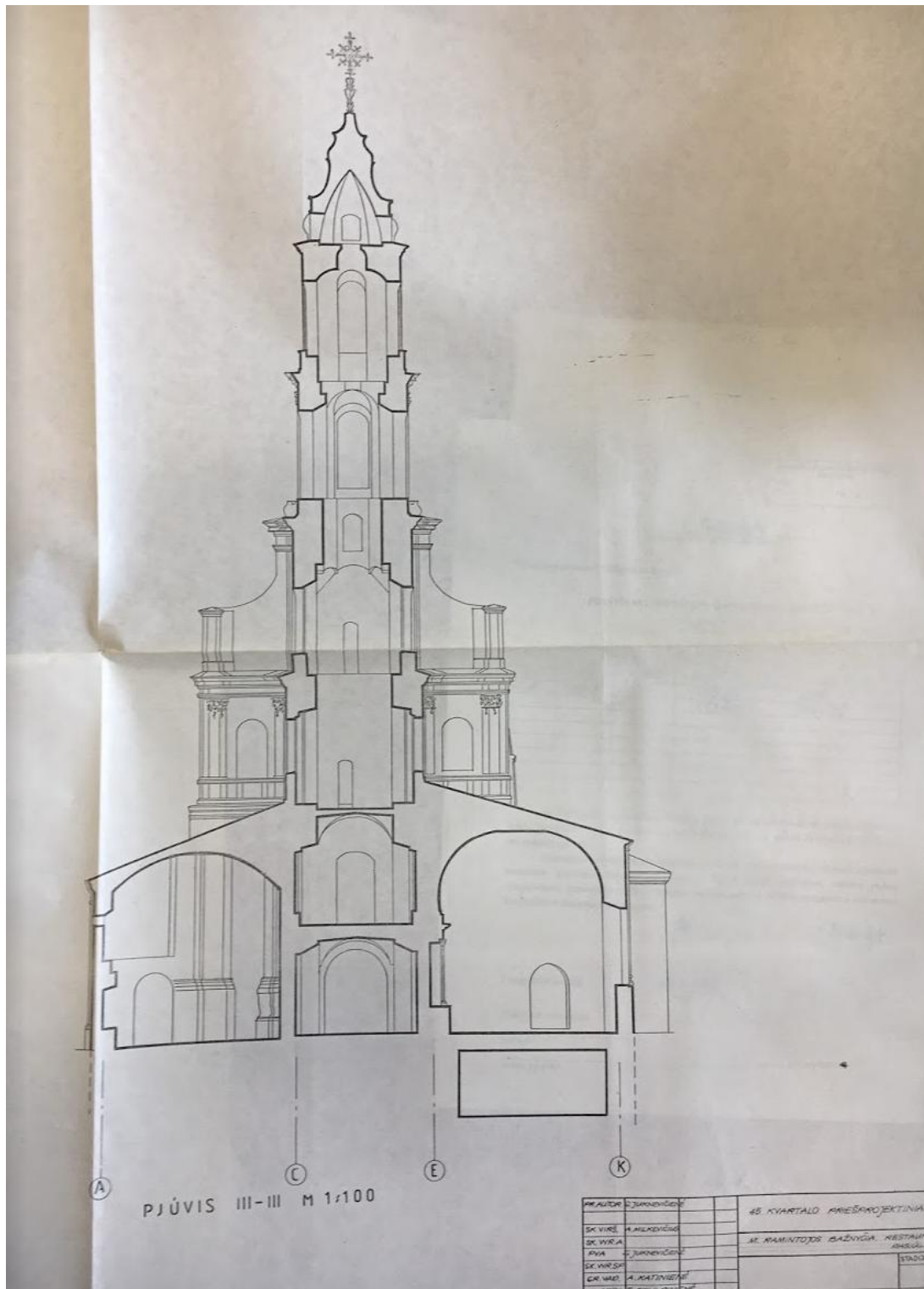
Pjūvis III
