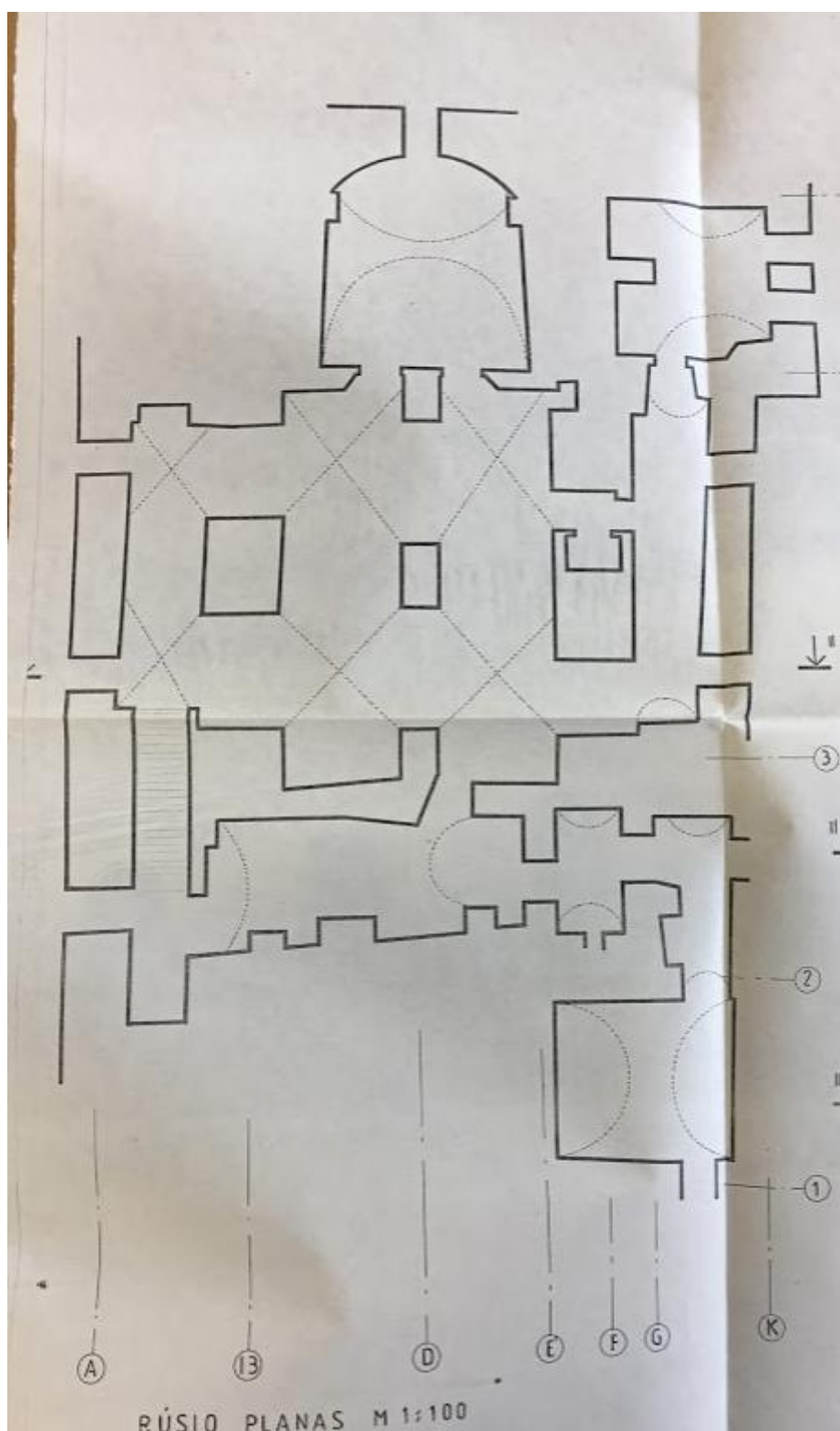
Rūsio planas
