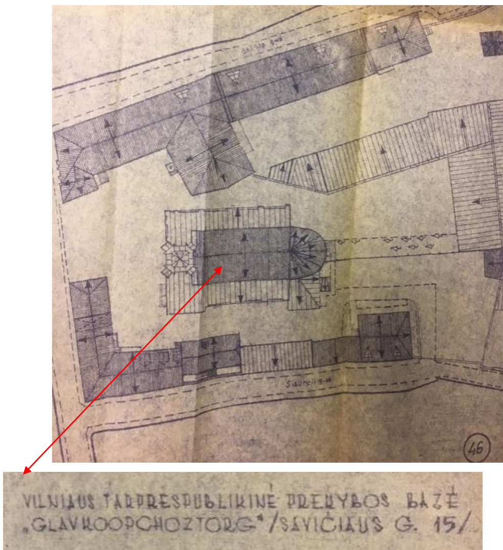
37. Stogų planas XX a. 8 deš.
