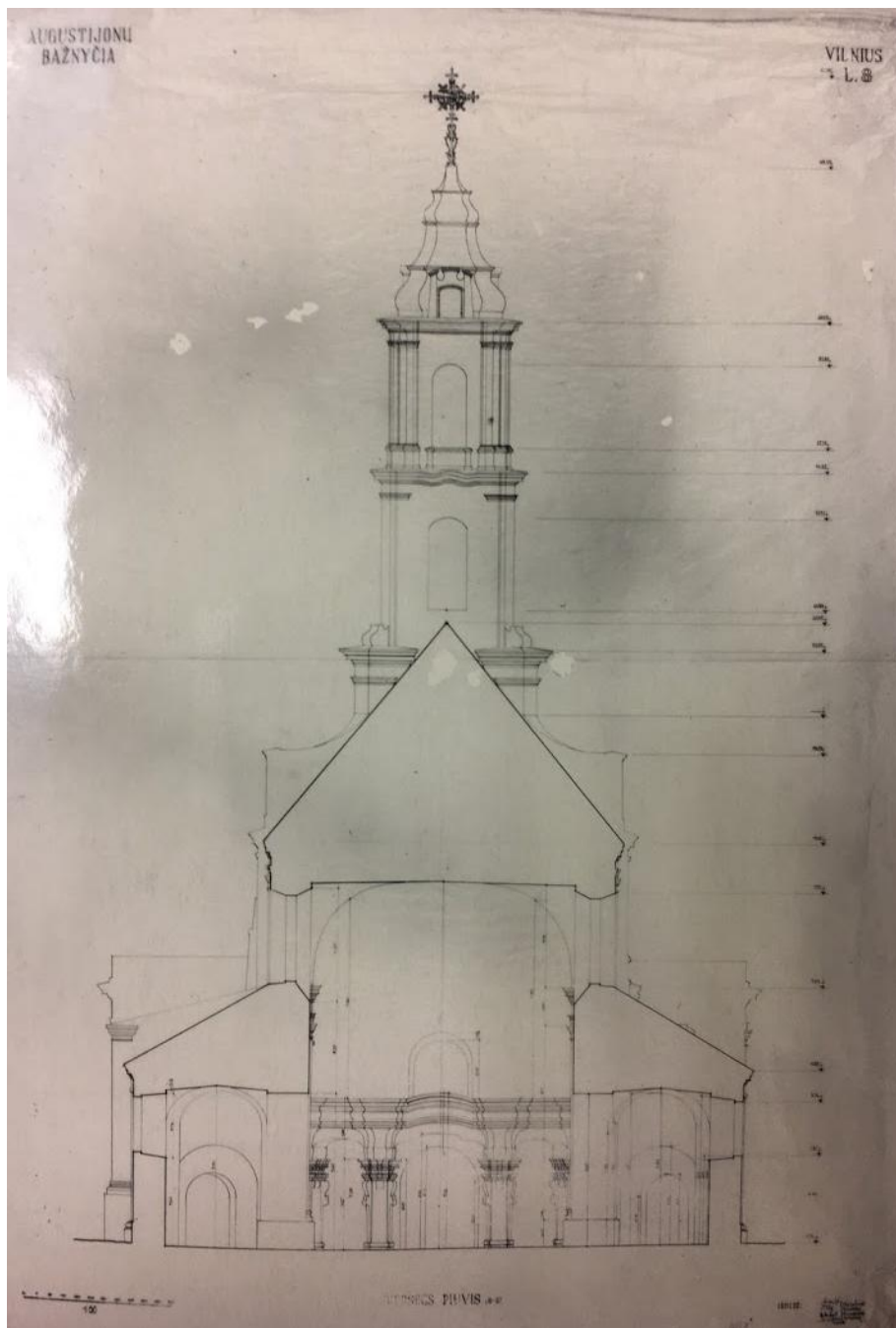
23. Išilginis pjūvis
