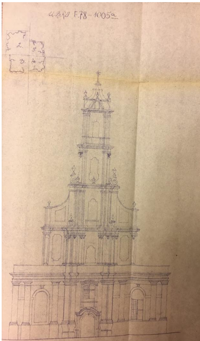
17. Apmatavimų brėžinys .1953 m. apmatavimai
