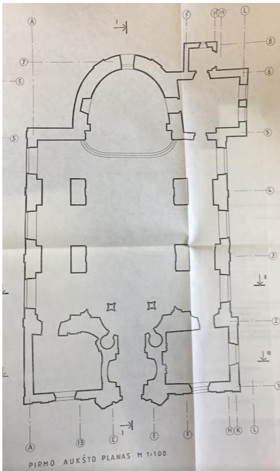
Pirmojo aukšto planas
