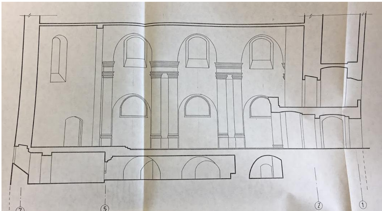
Išilginis pjūvis
