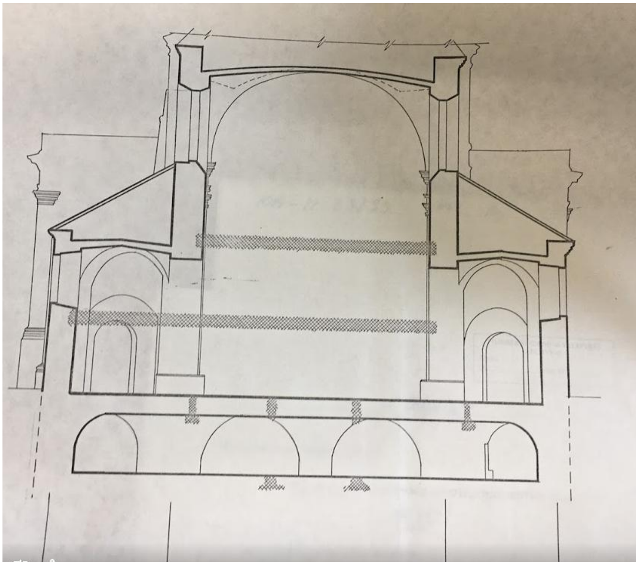
Pjūvis I
